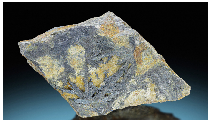
Stattliches Rauchquarz-Zepter, Kuhbergbruch, Neumühle, Thüringen, 10,5 x 5,8 x 4,6 cm (Foto links), Strahliger Antimonit (Stibnit) mit Quarz als Klufffüllung, 16 x 11,5 x 7,5 cm, beide Exponate Sammlung Museum für Naturkunde Gera.
